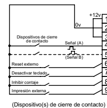
(Dispositivo(s) de cierre de contacto)
