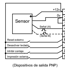
(Dispositivos de salida PNP)
