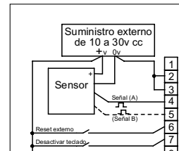
Uso ilustrado del suministro eléctrico externo (modo de generador).
