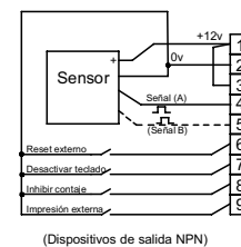
(Dispositivos de salida NPN)
