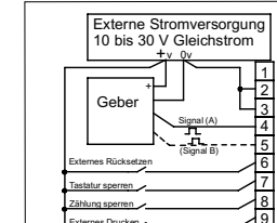
Externe Stromversorgung (Source Mode dargestellt)
