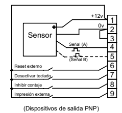
(Dispositivos de salida PNP)
