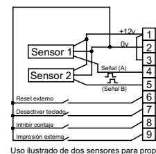
Uso ilustrado de dos sensores para proporción las señales A y B (modo de carga)
