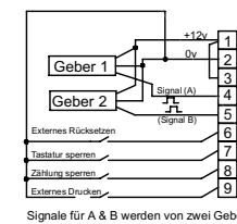
Signale für A & B werden von zwei Gebern bereitgestellt (Sink Mode dargestellt)
